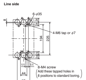
Load side
