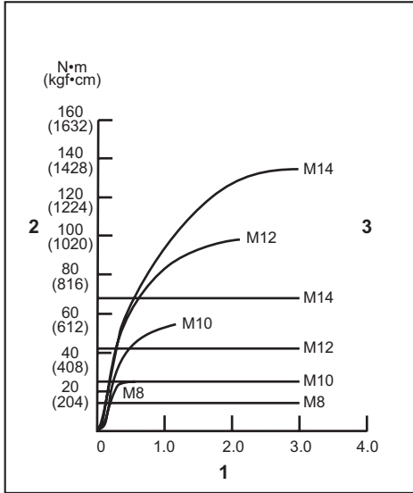
1. 紧固时间(秒) 2. 紧固转矩 3. 紧固转矩视各个螺栓的直径不同而异
