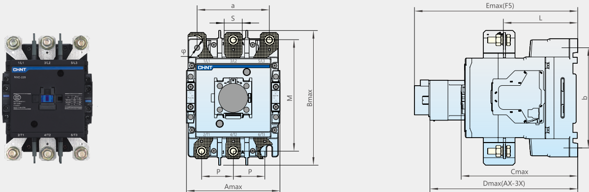
NXC-120~225 外形尺寸与安装尺寸
