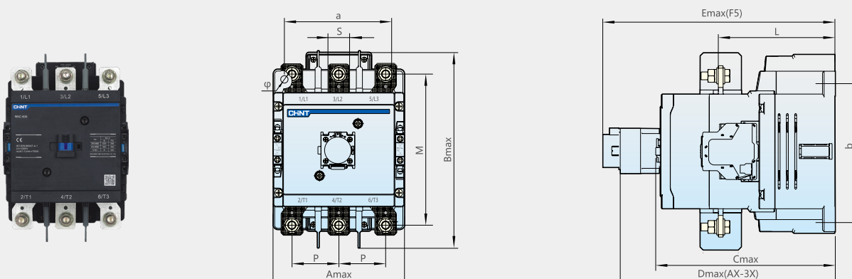
NXC-500~630 外形尺寸与安装尺寸
