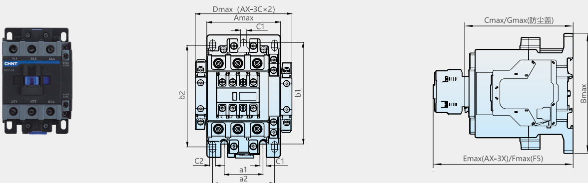
NXC-40~100 外形尺寸与安装尺寸
