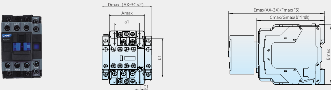
NXC-06~38 外形尺寸与安装尺寸
