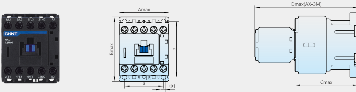
NXC-06M~12M 外形尺寸与安装尺寸
