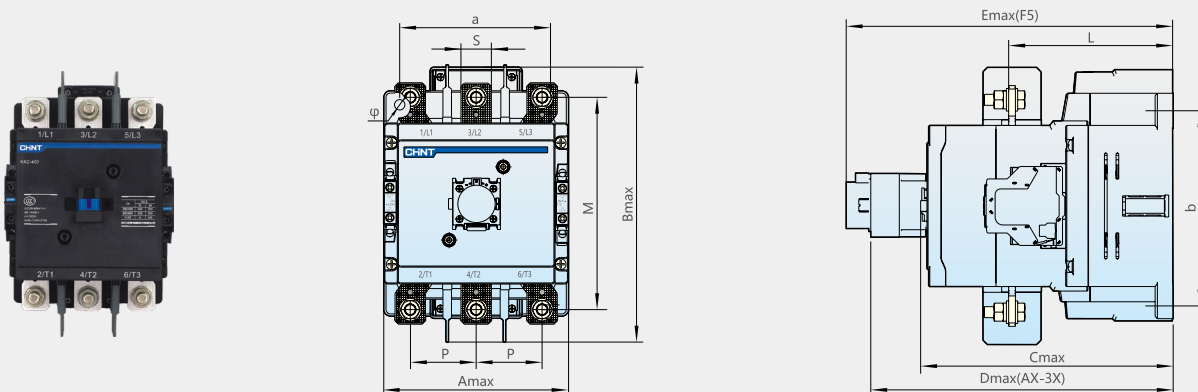
NXC-265~400 外形尺寸与安装尺寸
